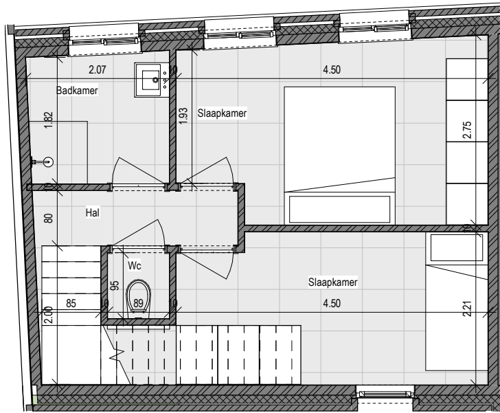
Eerste verdieping
