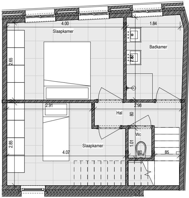
Eerste verdieping
