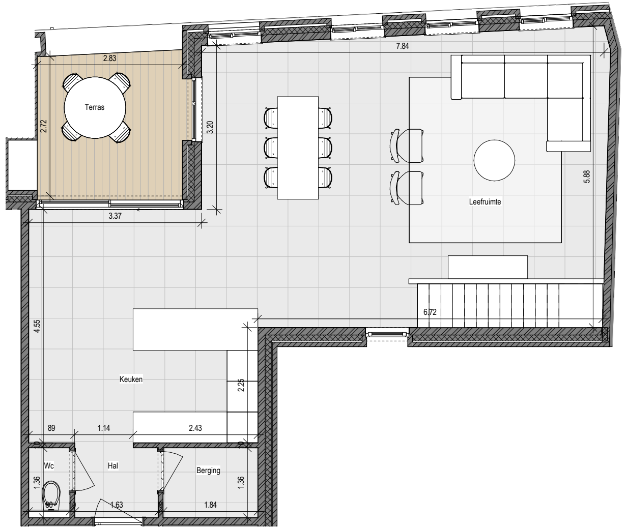
Tweede verdieping
