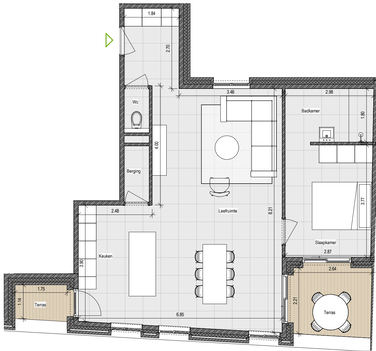
Tweede verdieping 1 : 75
